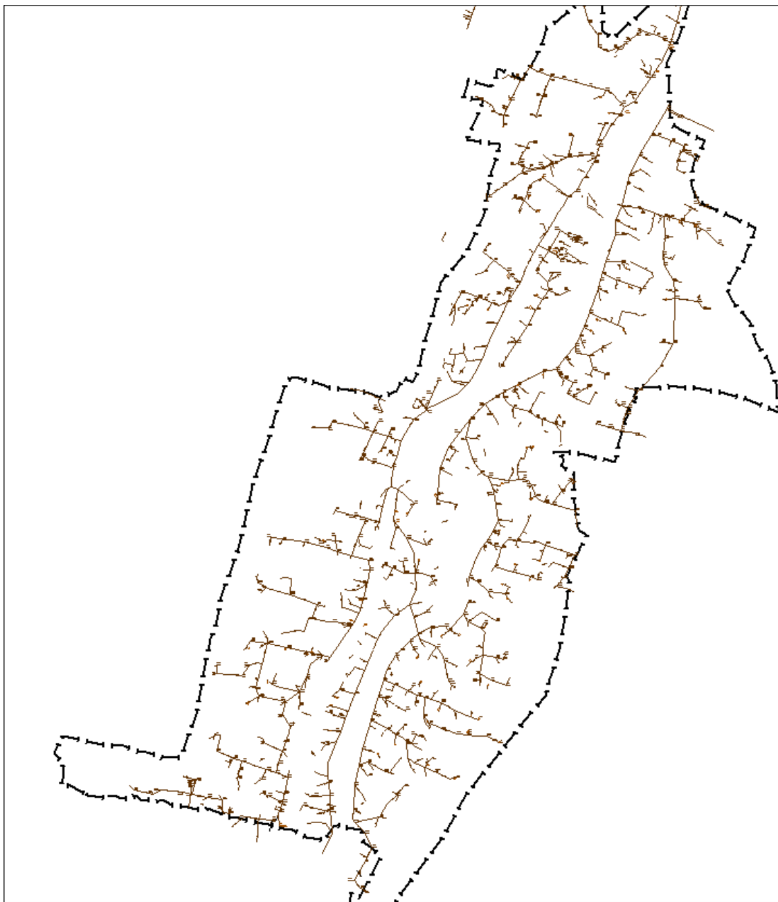
Ryc. Kanalizacja sanitarna na terenie Posady Górnej
